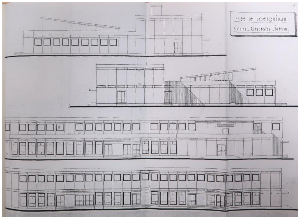
Cuisine - réfectoire- infirmerie. Élévations.
