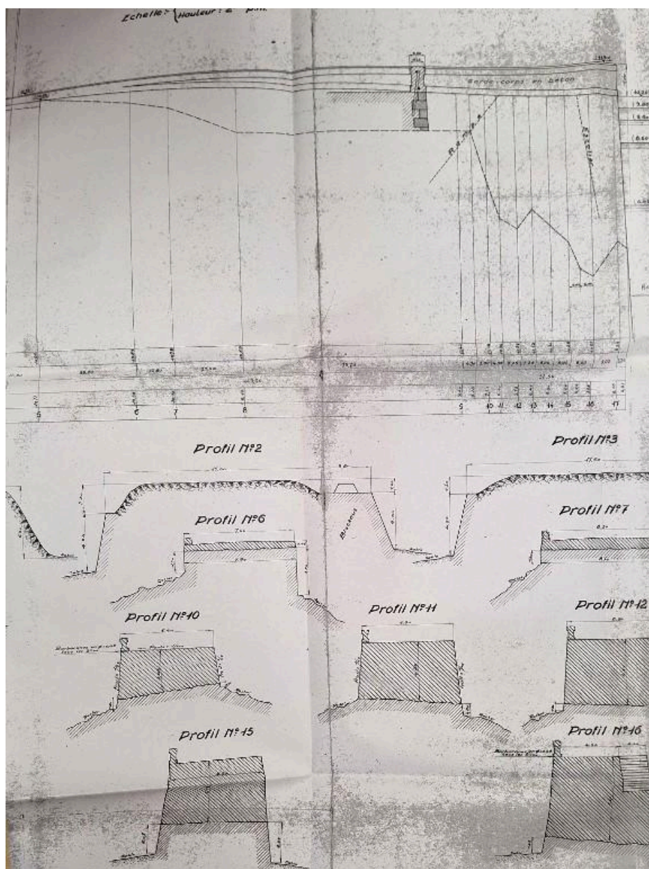
Coupe, profils de l'ouvrage de Pen ar Vil, juillet 1947
