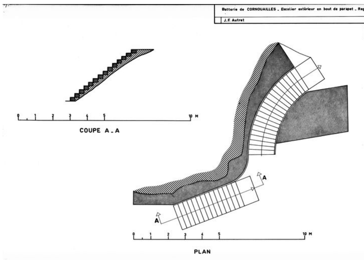
Plan et coupe A-A de l'escalier extérieur de la grande batterie de Cornouaille
