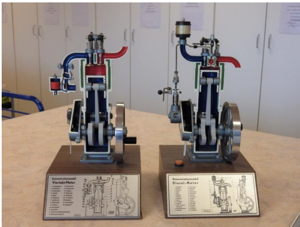
Modèle de moteur à quatre temps et modèle de moteur diesel - Chaleur (Höhm, 1950-1975)
