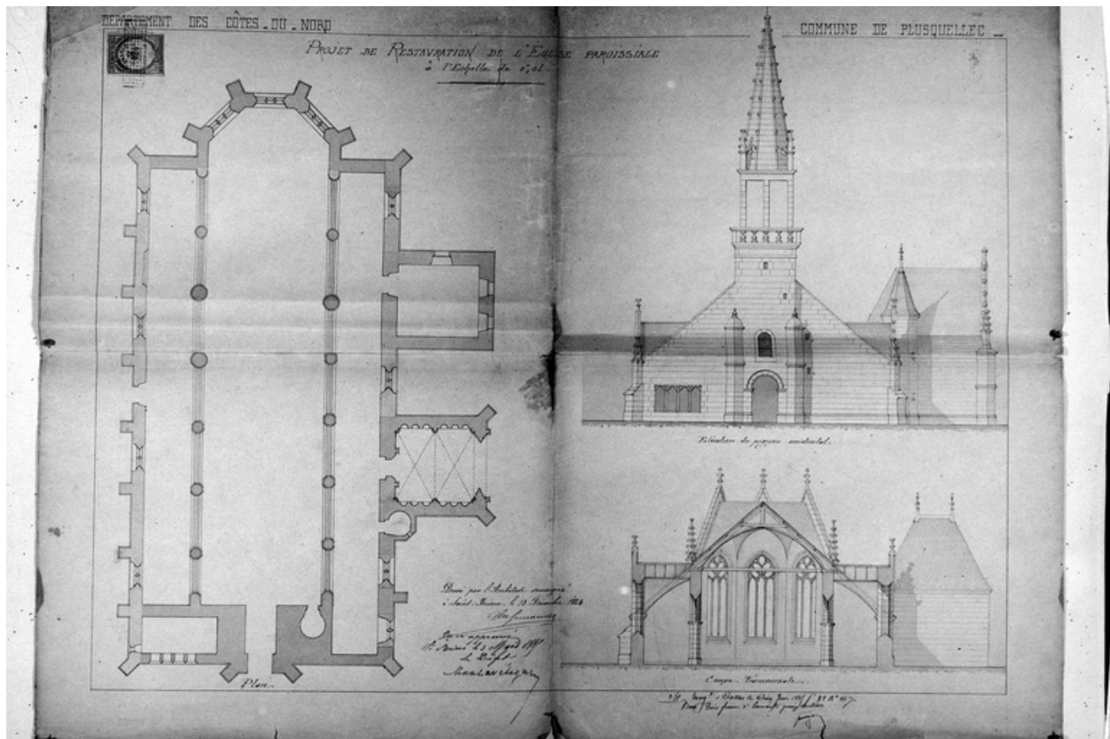
Projet de restauration (plan-coupe transversale et élévation de la façade ouest)
