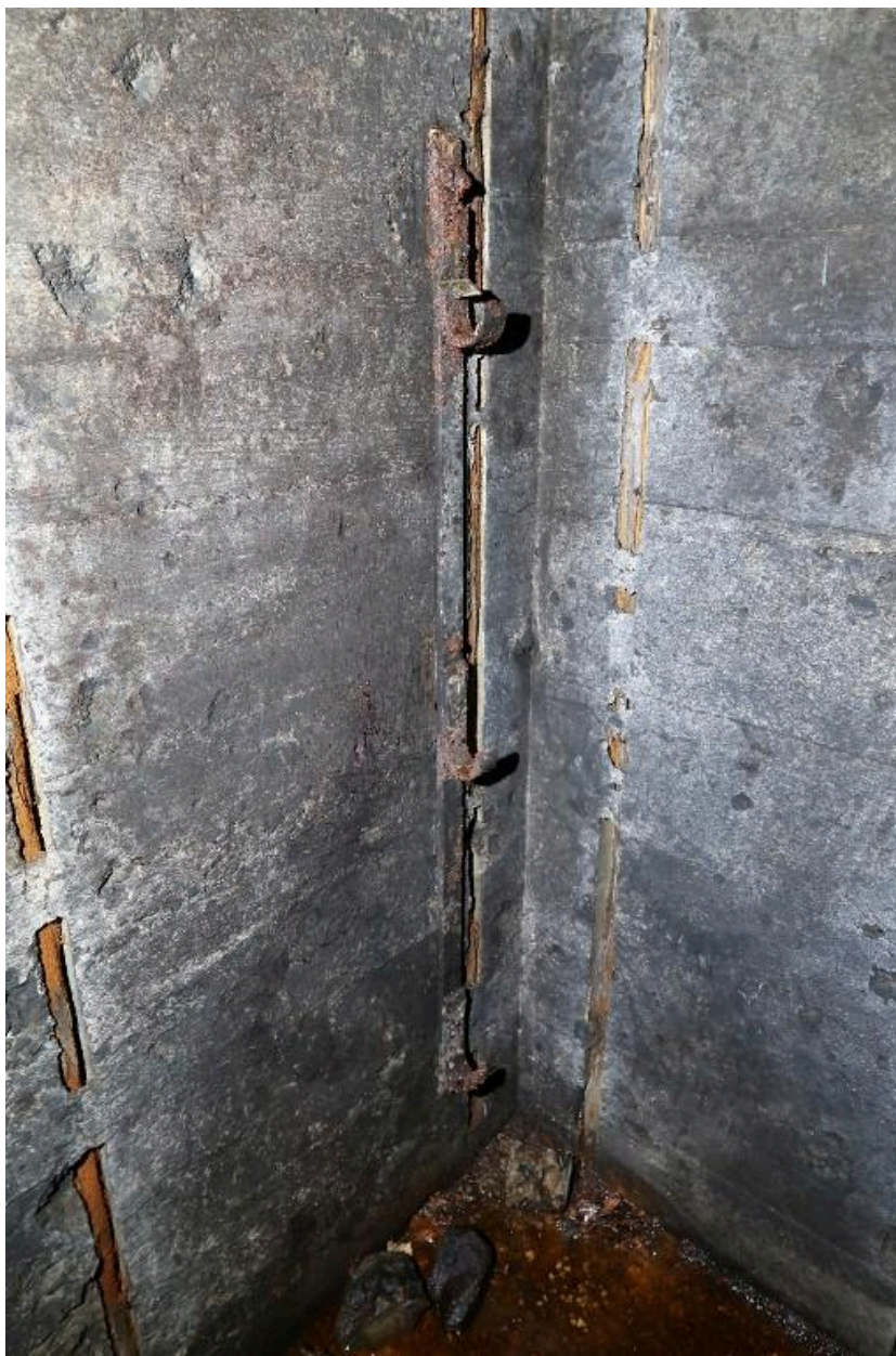
Vue intérieure : support vertical pour couchettes tubulaires rabattables sur trois niveaux
