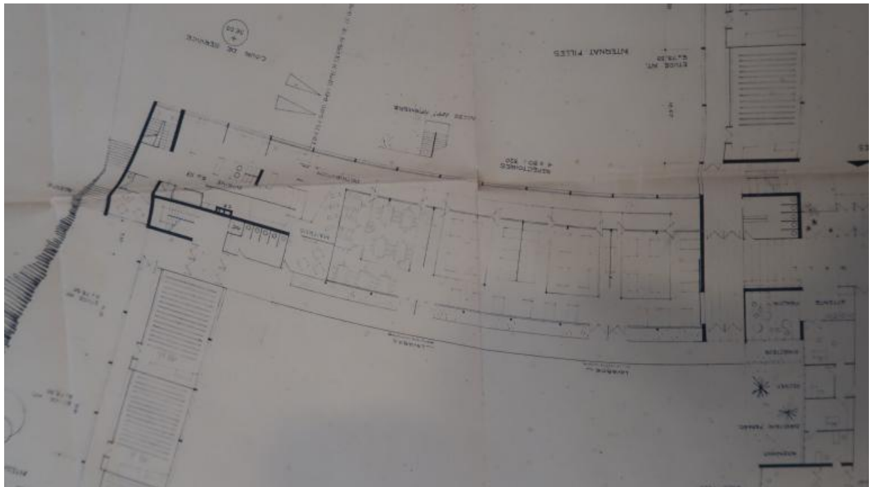
Plan des réfectoires et cuisine. Raymond Lopez, architecte, 1956.
