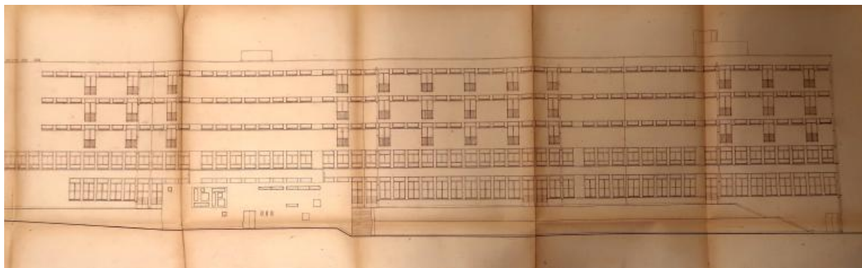
Internat - Bâtiment A. Façade est. Yves Moignet, architecte, 1960.
