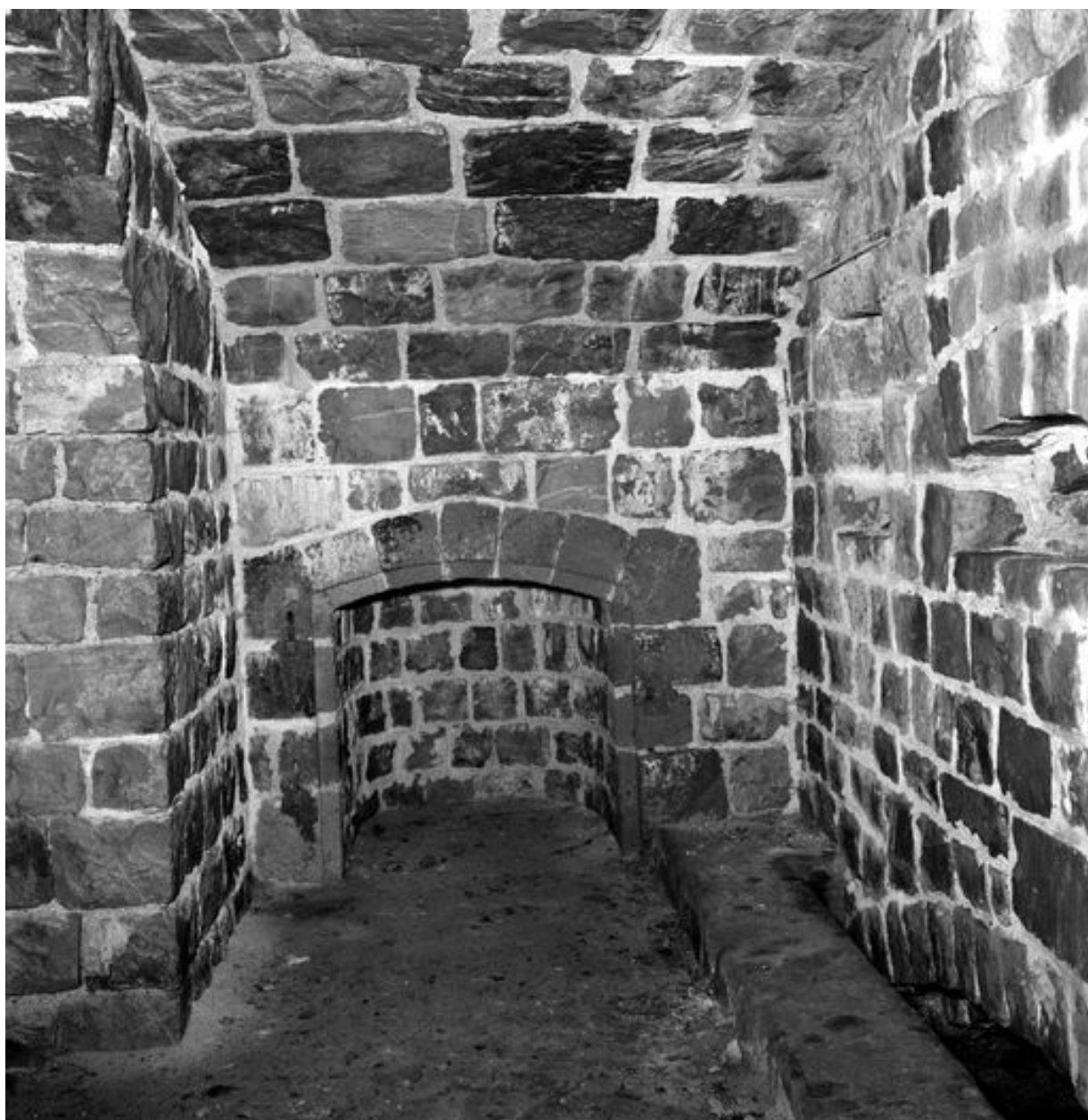
Vue du réduit de Landaoudec en 1969 : caponnière, extrémité gauche de la galerie enveloppe
