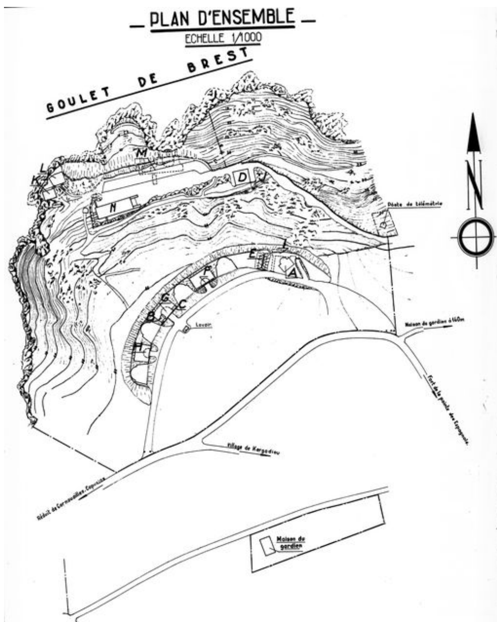
Plan d'ensemble au 1/1000 des batteries Robert
