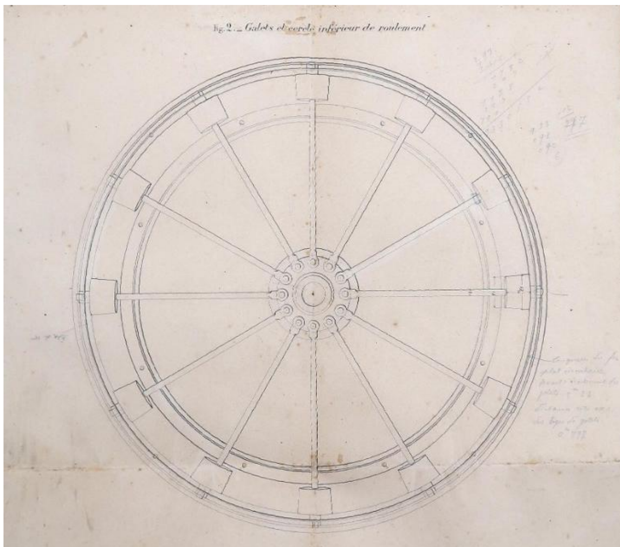
Galets et cercle intérieur du roulement (14 avril 1890)
