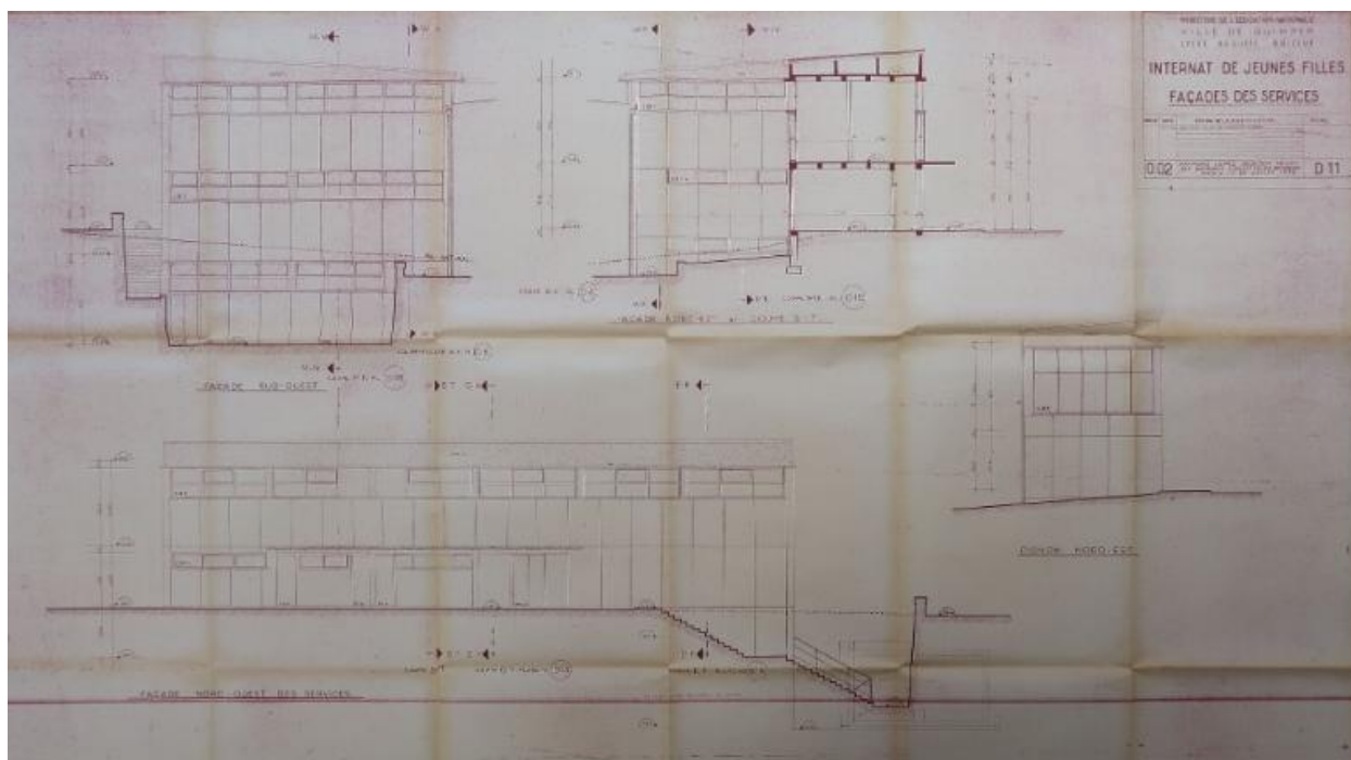
Internat de jeunes filles. Façade des services. Raymond Lopez, architecte, 1952.
