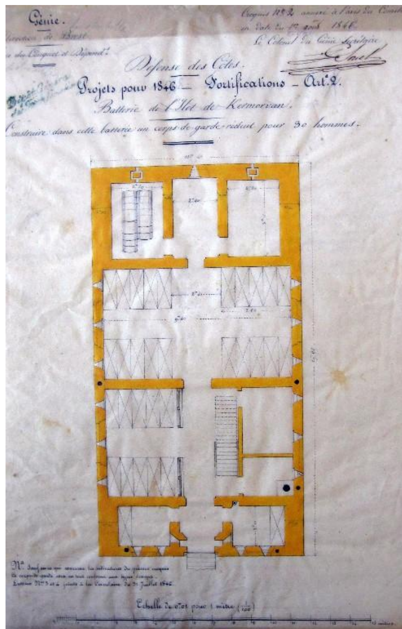
Plan du corps de garde crénelé pour 30 hommes pour la batterie de l'Îlet de Kermorvan, projet pour 1846
