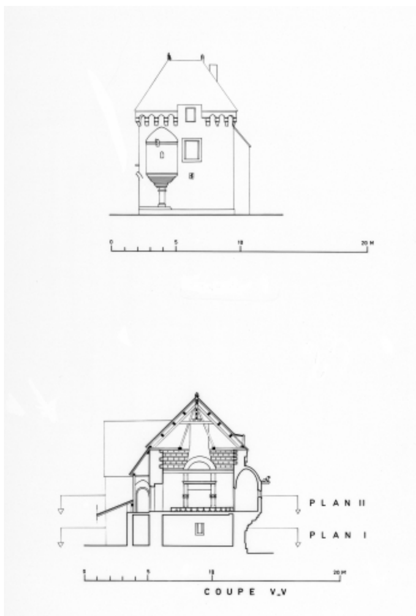
Manoir de la Ville Blanche (Canihuel) : Elévation sud, coupe
