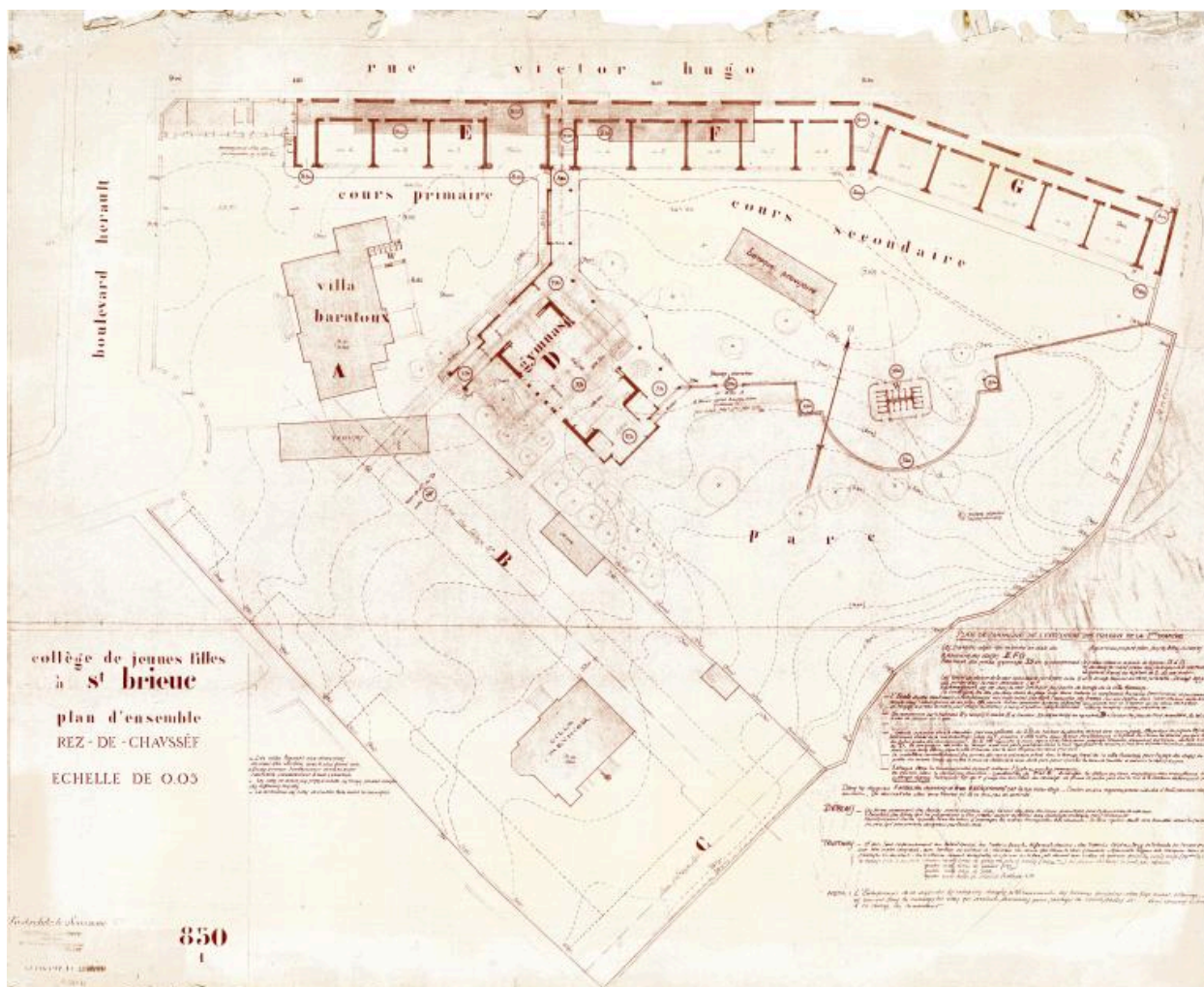
Plan masse, 1934.
