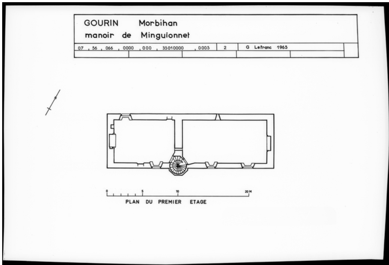
Plan du premier étage.
