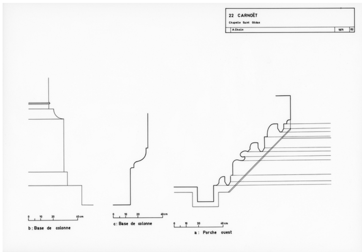
Profil des moulures, base de colonne, porche ouest
