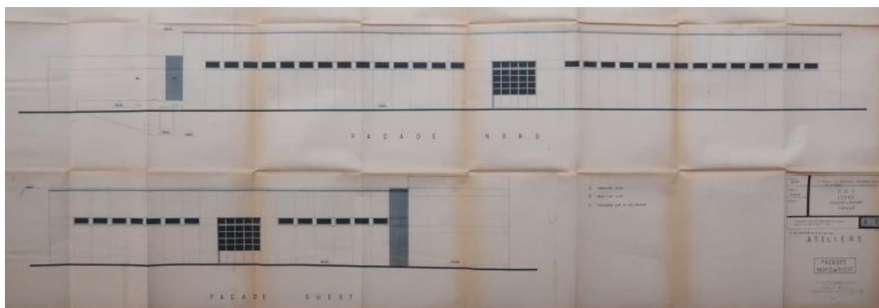
Ateliers, façades nord et ouest. Hervé Péron et Alexandre Weisbein, architectes, 1964.
