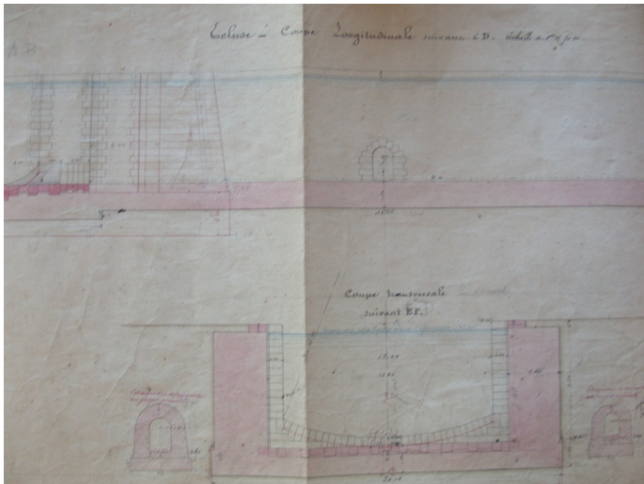
Dessin : coupe longitudinale d'un vantail de la 1ère écluse, 1875 (AD 22)
