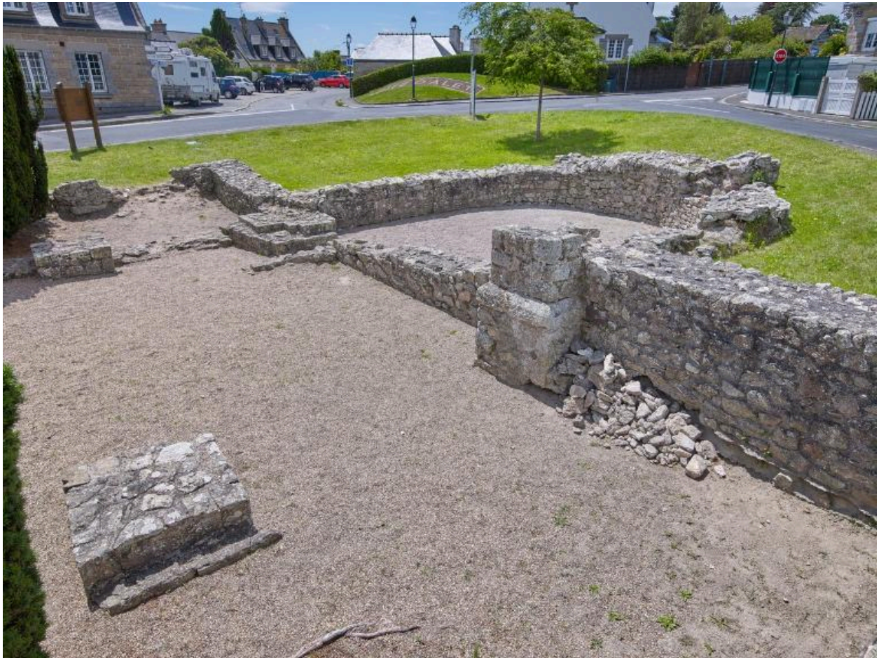
Vue de détail de l'abside occidentale avec les bases de piles de la nef
