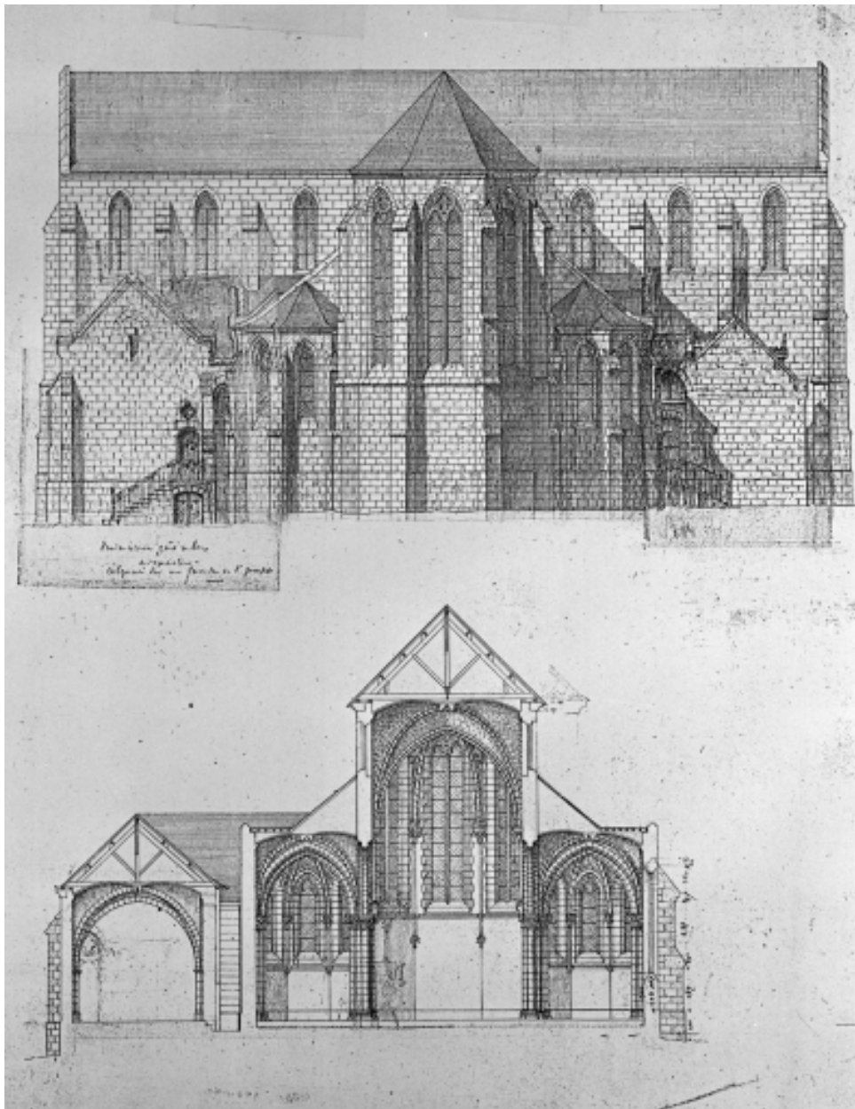
Elévation de la façade absidiale
