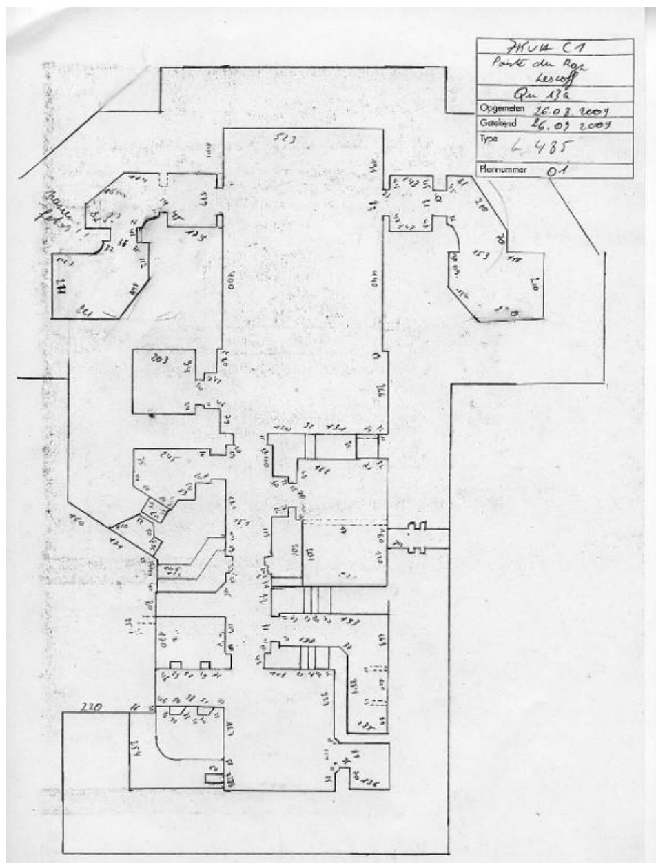
Plan du bunker de type L 485 de (dessin : Dirk Peeters, 2009)
