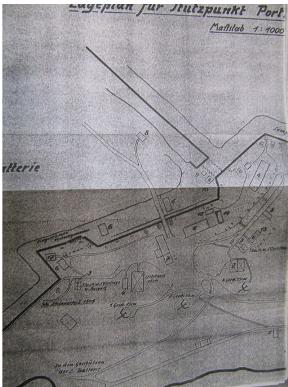
Extrait du plan allemand de l'ensemble fortifié du Portzic
