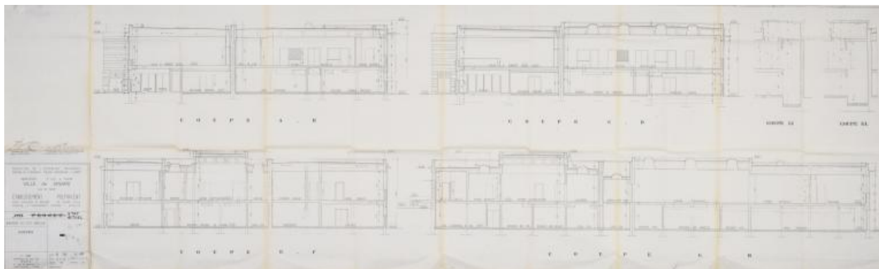
Coupes des ateliers ("bâtiment n°1 C.E.T. hôtelier"). Patrice Simon, architecte, 25/09/1970.
