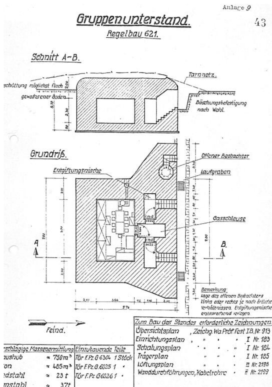
Plan-type d'un bunker - abri de type 621 (Gruppenunterstand für 10 Mann)
