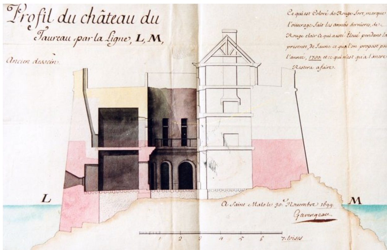
Coupe du fort par la ligne L M, fait à Saint-Malo le 30 novembre 1699 par Garengau
