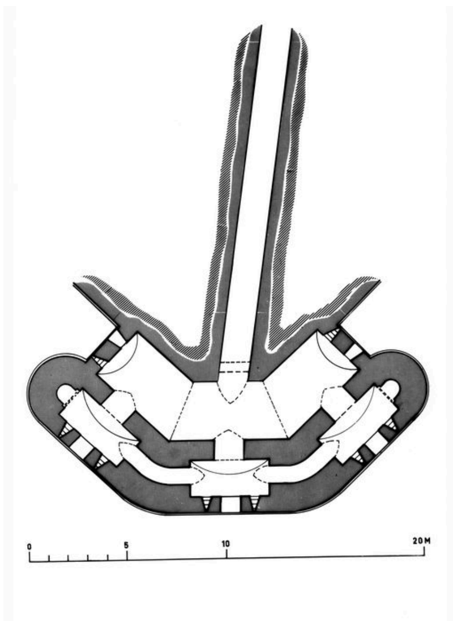
Plan, détail du réduit de Landaoudec, Crozon (Lecoq)
