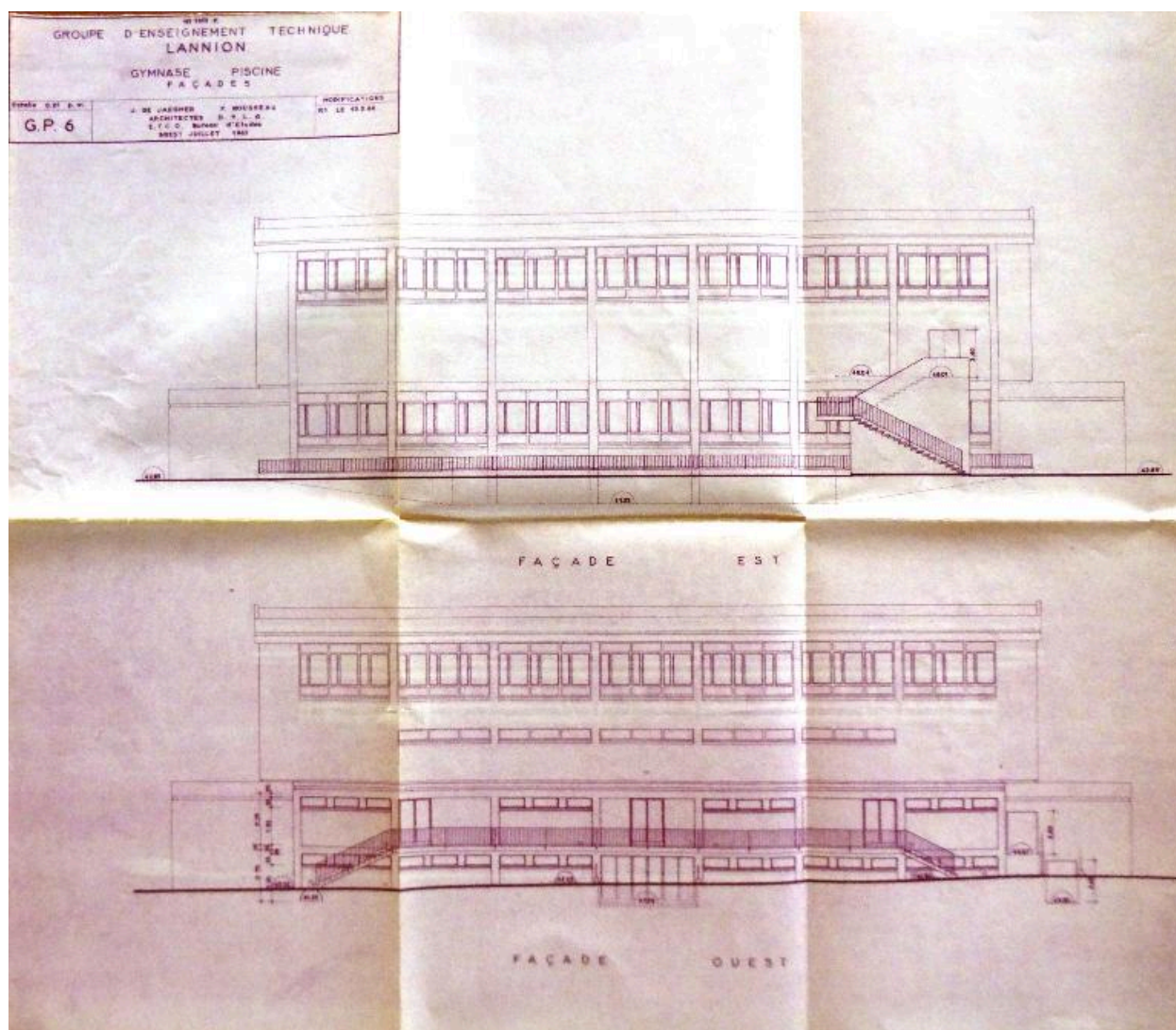
Façades est et ouest du gymnase-piscine
