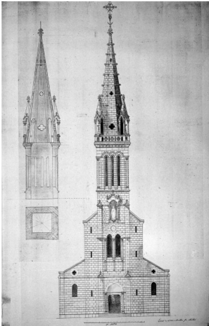
Plan de la façade d'entrée.
