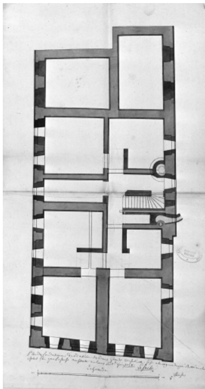
Plan des fondations par Le Saché, 1738 (A. D. Ille-et-Vilaine)
