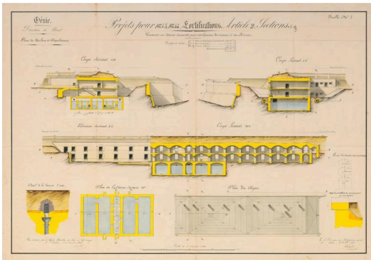
Place de Quéléren et dépendances, projets pour 1853-1854 : plan, élévations et coupes de la caserne casematée pour 635 hommes du fort de Quéléren, des cuisines et des latrines, 22 décembre 1852
