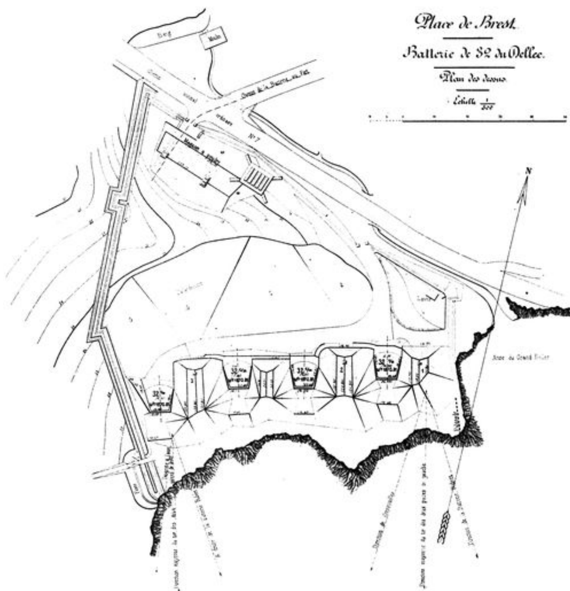
Plan de de la batterie de 32 cm du Dellec
