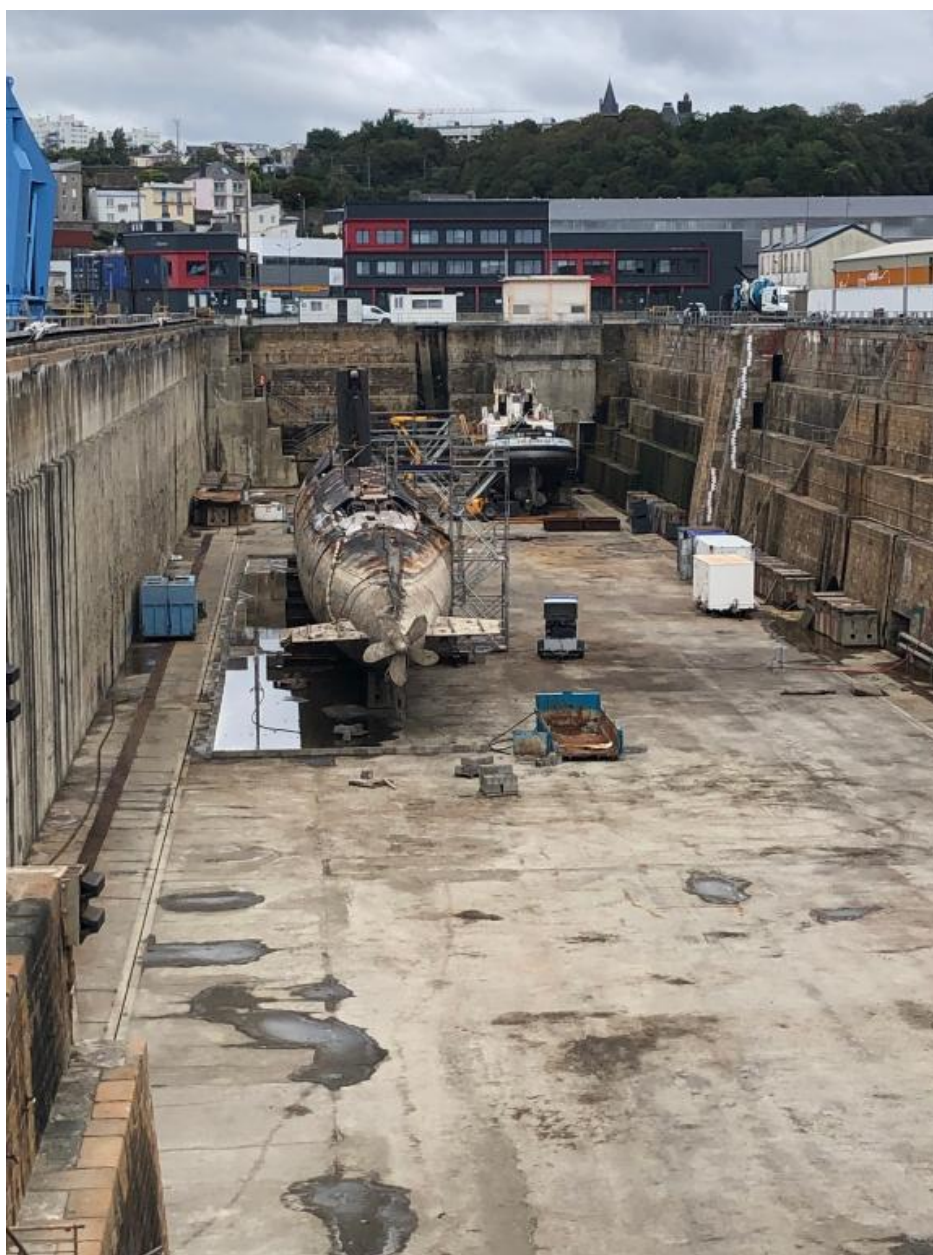
La coque de l'Agosta dans la forme de radoub n° 1 du port de Brest, 18 août 2021
