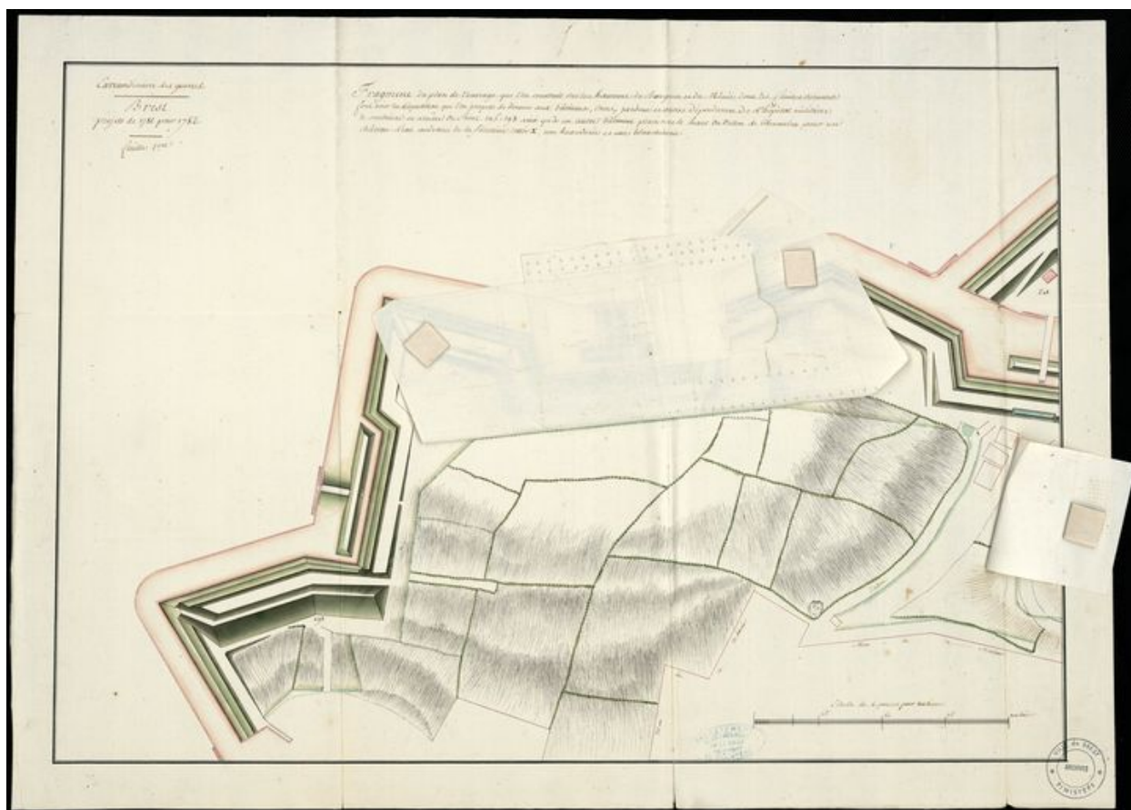
Projet d'hôpital militaire sur les hauteurs du Bouguen et du Menès à Brest, projet de 1781 pour 1782 : plan d'ensemble
