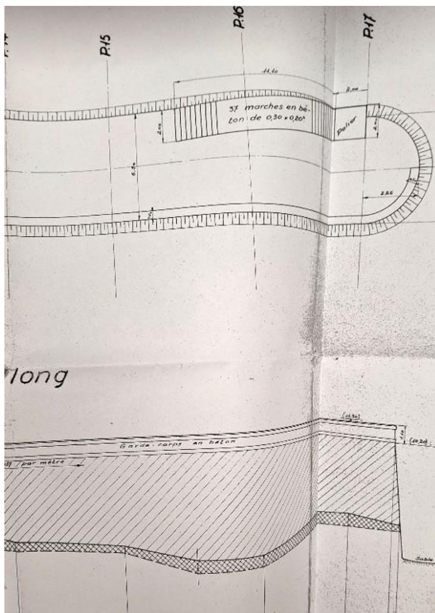
Coupe, profils de l'ouvrage de Pen ar Vil, juillet 1947
