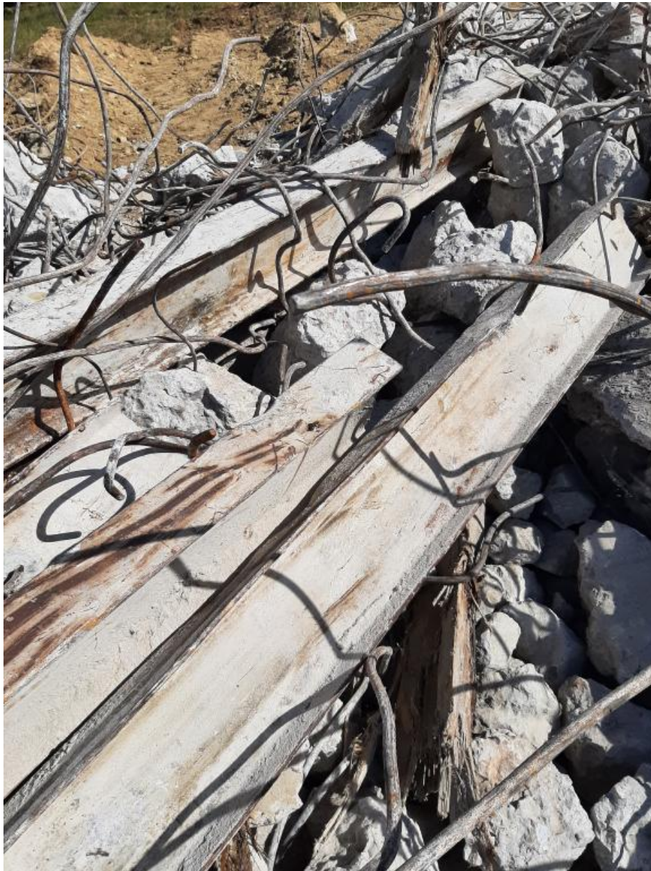
Vue de la déconstruction : matériaux de la dalle de couverture et des murs périphériques (25 septembre 2022)
