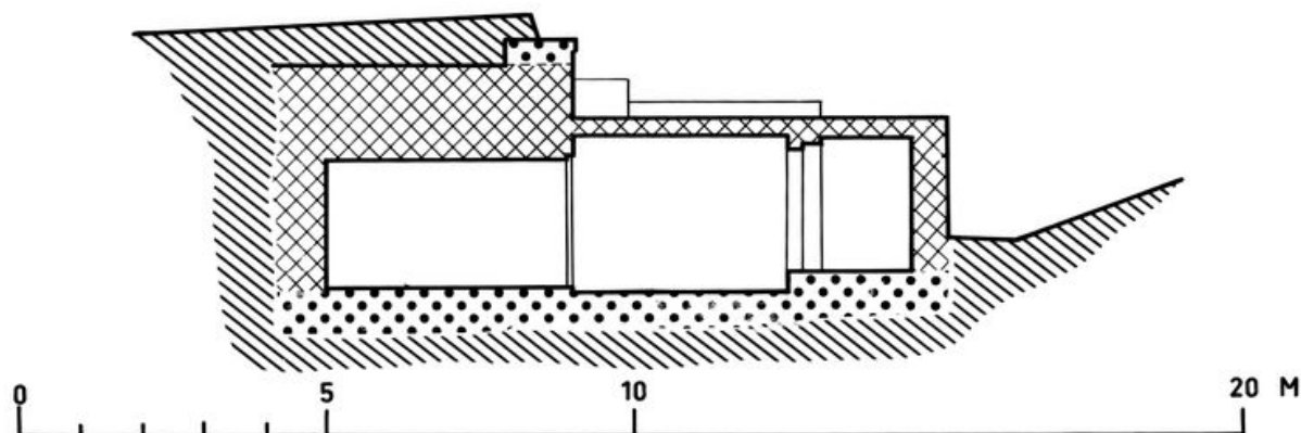
COUPE A - A
