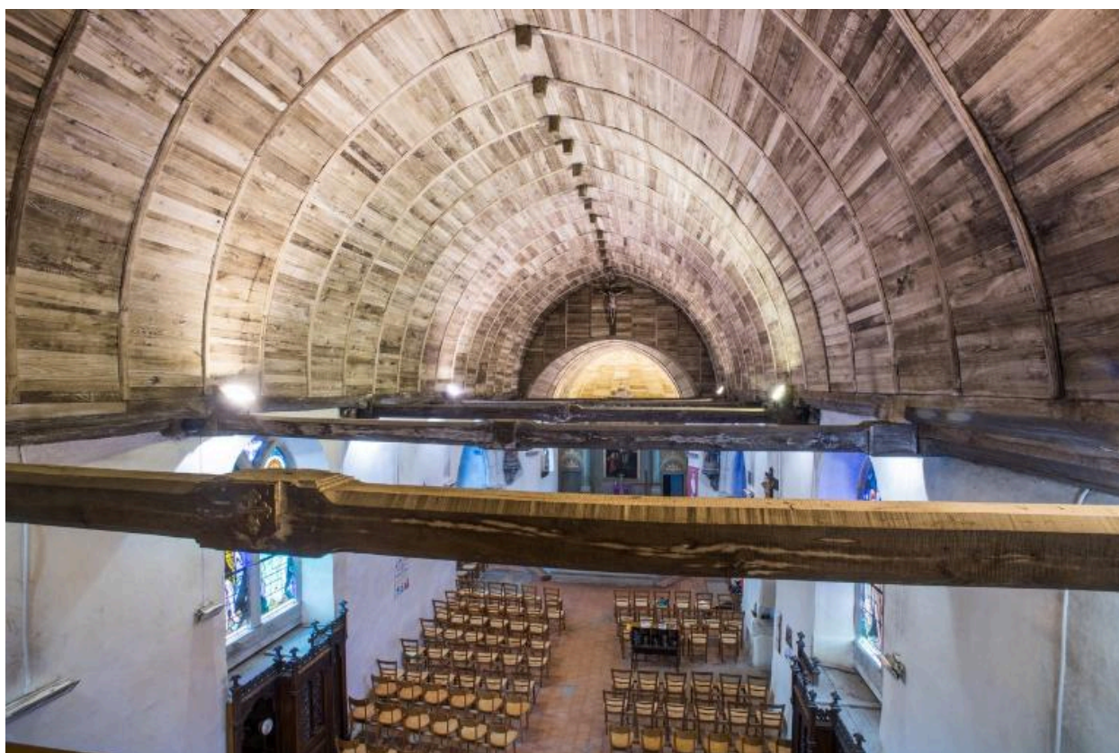
Vue de la voûte lambrissée en chêne en plein cintre depuis l'orgue (vue depuis l'Ouest)
