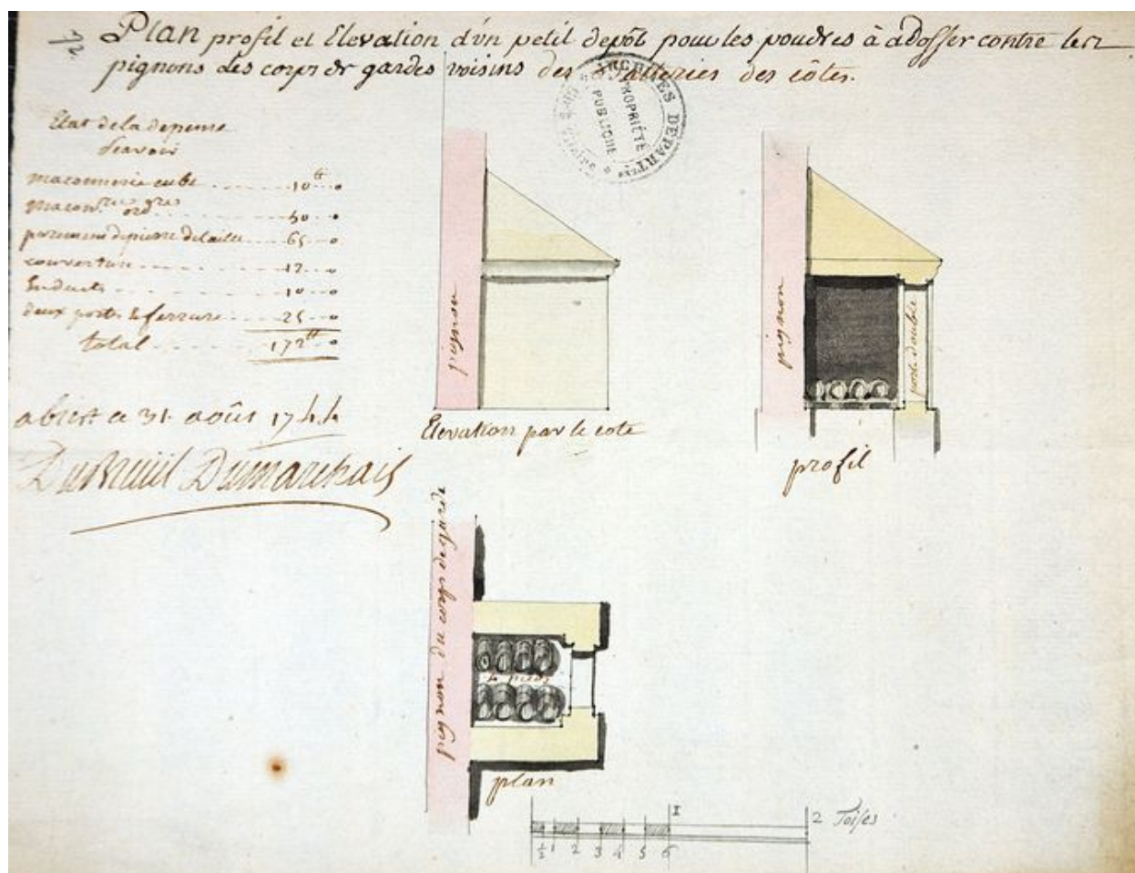
Elévation, plan et profil d'un petit dépôt pour les poudres adossé contre les pignons des corps de garde voisins des batteries de côtes, fait à Brest le 31 août 1744 par Dubreuil Dumarchais
