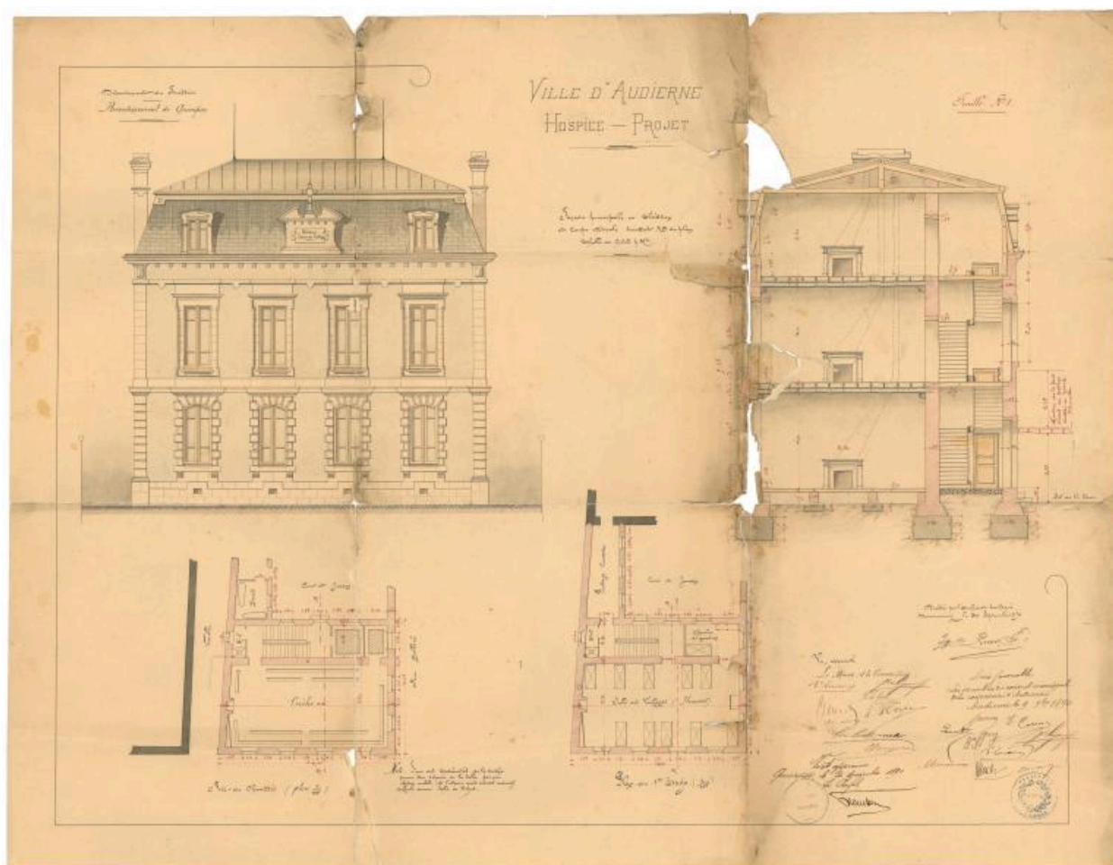
Plans élaborés par Ruer en 1890 : élévation, coupe et plans au sol.
