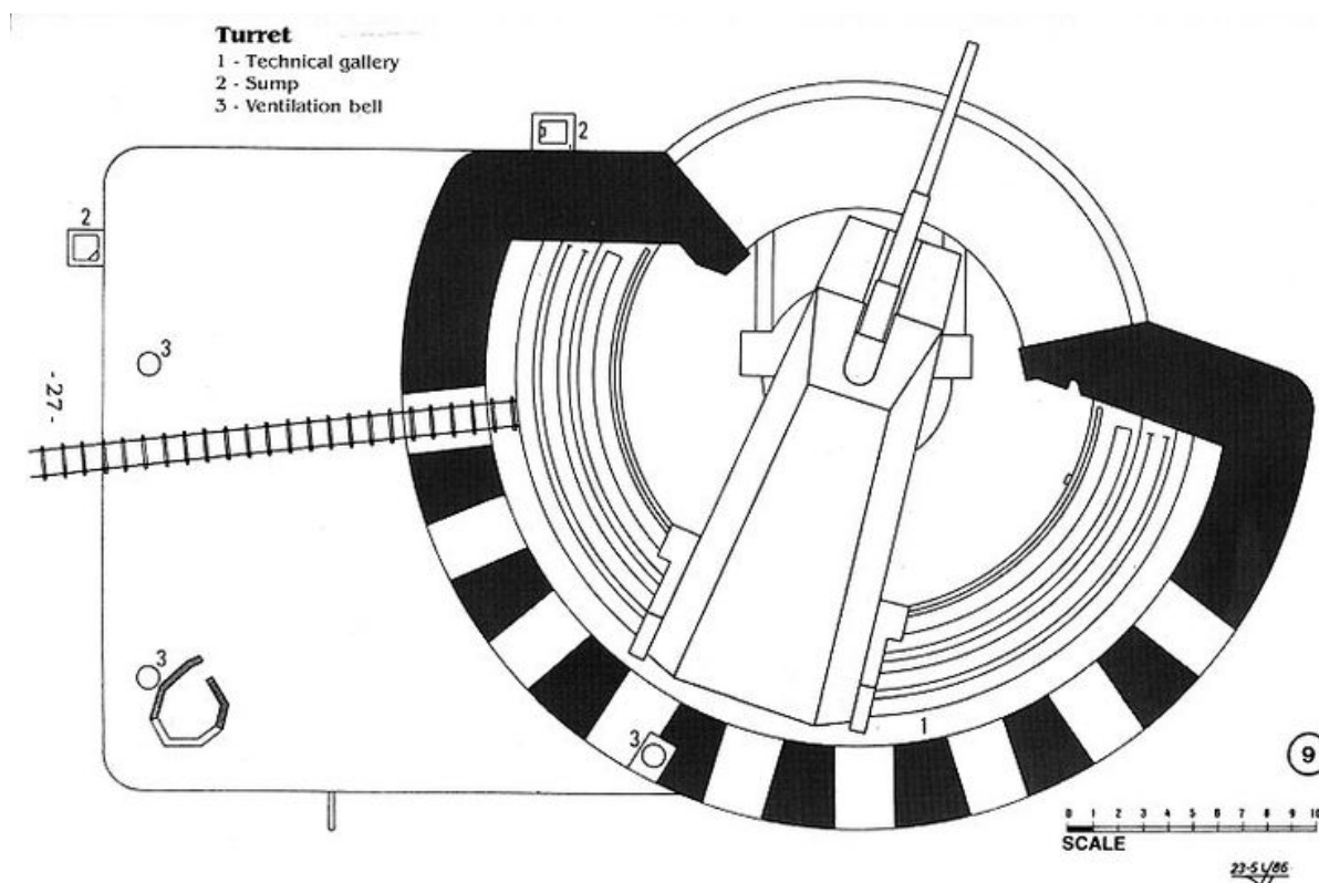
Plan du niveau +1 d'une des casemates de la batterie Todt (Pas-de-Calais). Dessin Yannick Delefosse
