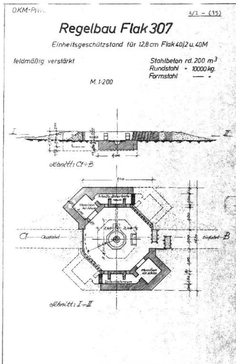
Plan et coupe d'un bunker - cuve de type FI 307 (Einheitsgeschützstand für 12,8cm Flak 40)
