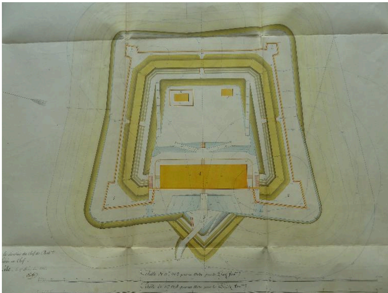
1 VH 292. Place de Belle-Ile, feuille des projets extraordinaires pour 1847, fort central de l'Île d'Hoedic, 17 décembre 1846.
