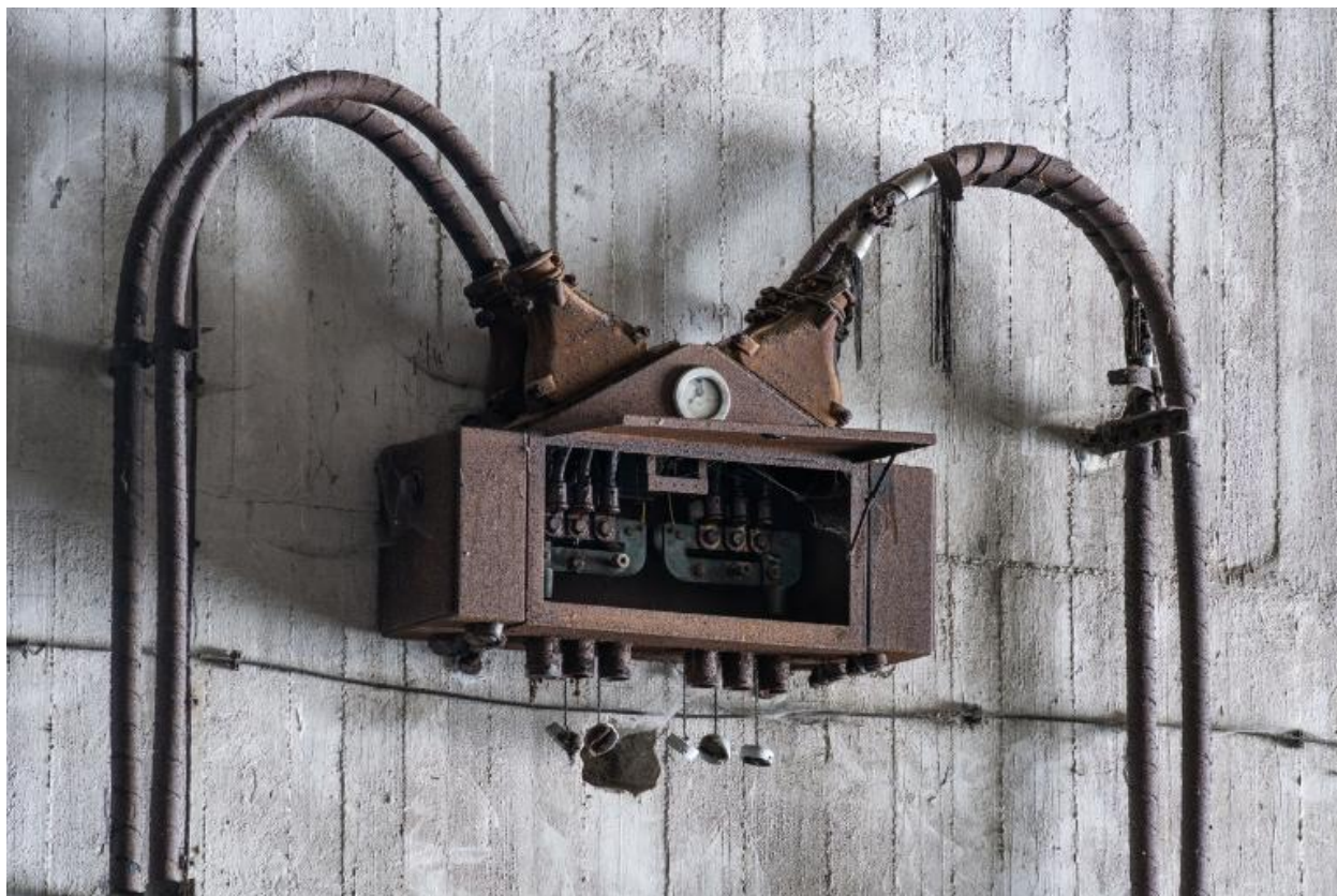
Vue d'un boîtier de connexion électrique avec voltmètre (quatre arrivées de câble pour six sorties)
