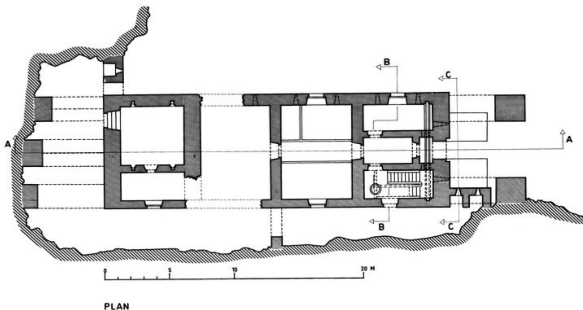
Plan de la caserne défensive
