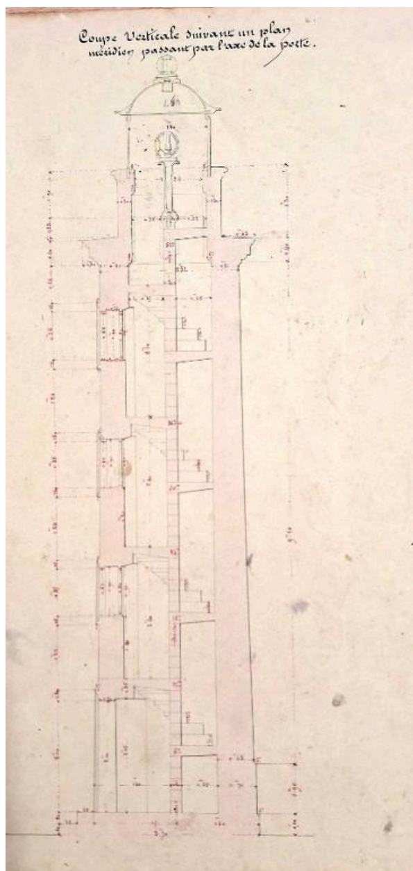
Coupe verticale du phare de la pointe de l'Aigle (29 novembre 1851)
