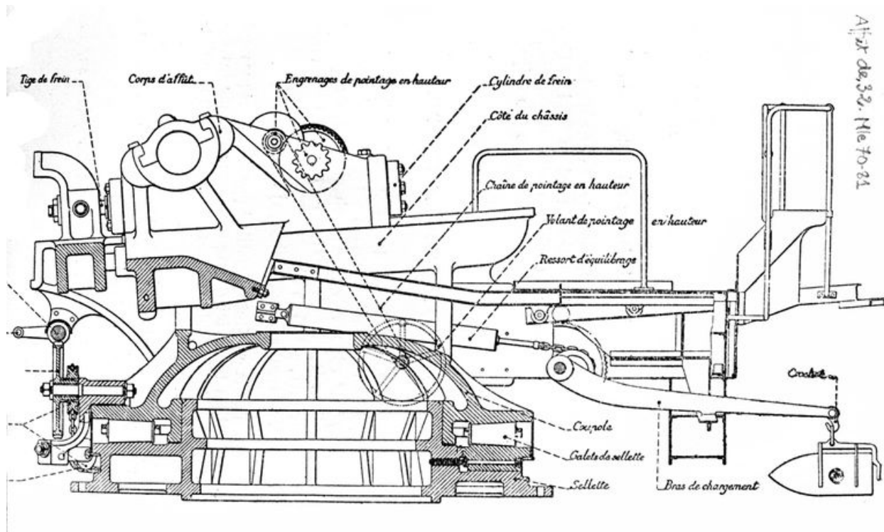
Plan détaillé d'un affût de 32 cm modèle 1870-1881
