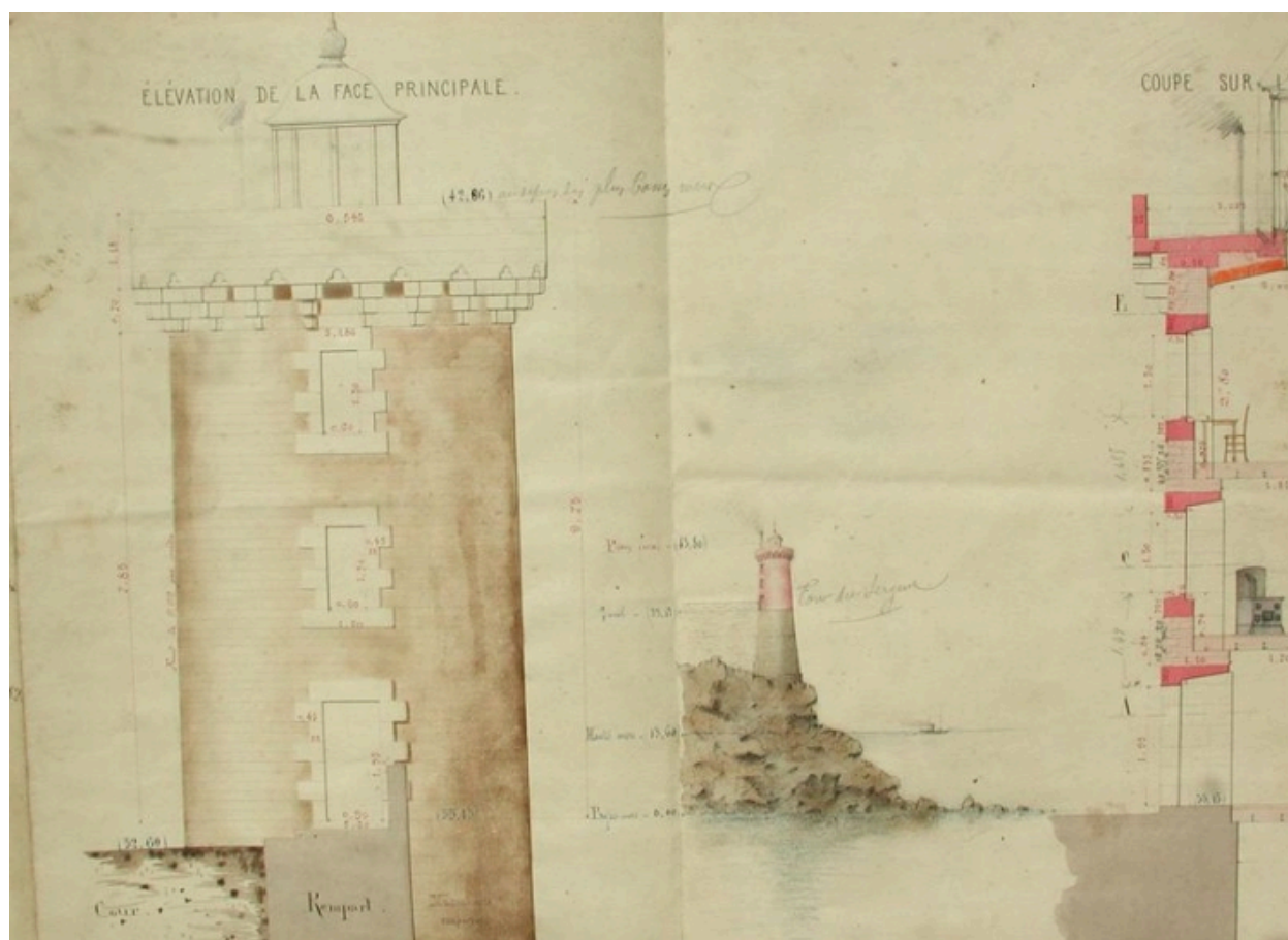
Projet de phare en 1882 à Fort-La-Latte : élévation de la face principale (AD 22)
