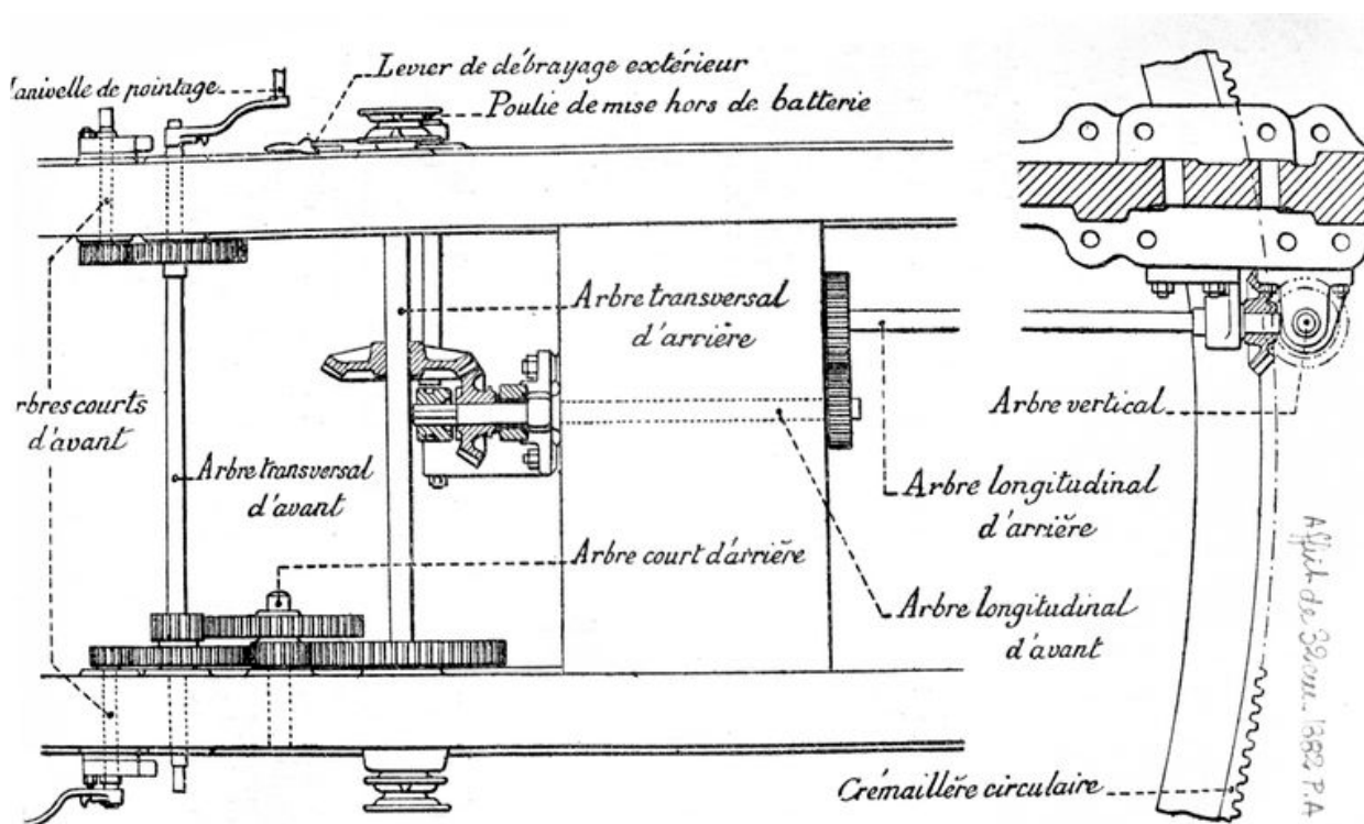
Plan détaillé d'un affût modèle 1882 PA pour canon de 32 cm
