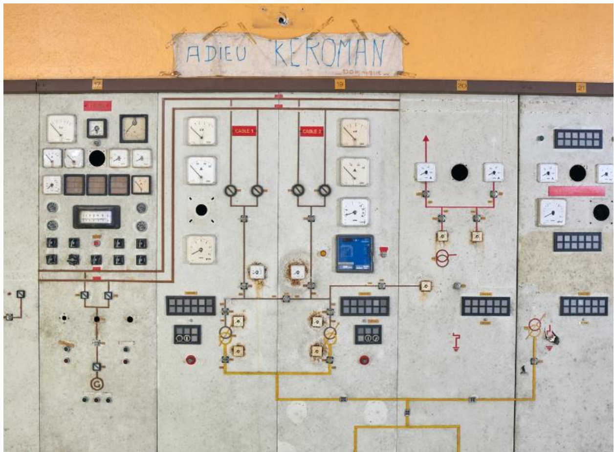
Vue de la salle de commande de la centrale électrique : tableaux n° 17 (G[rroupe] E[lectrogène] "DUVANT") , 18, 19, 20 et 21. Accochée au mur, banderole sur laquelle on peut lire "Adieu Keroman - Dominique"
